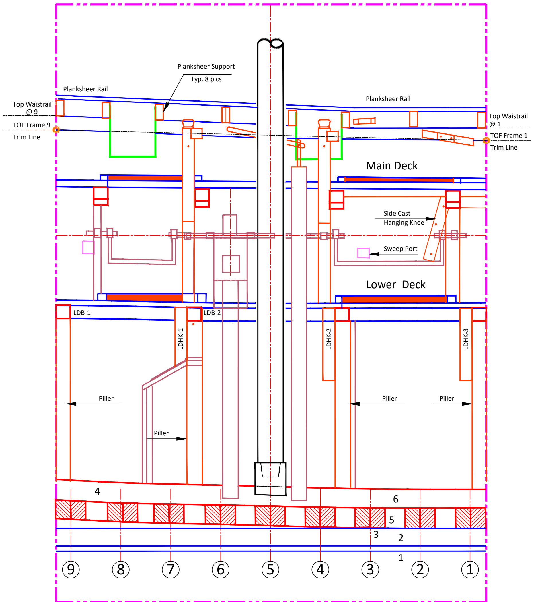
Longitudinal Section 1:32
