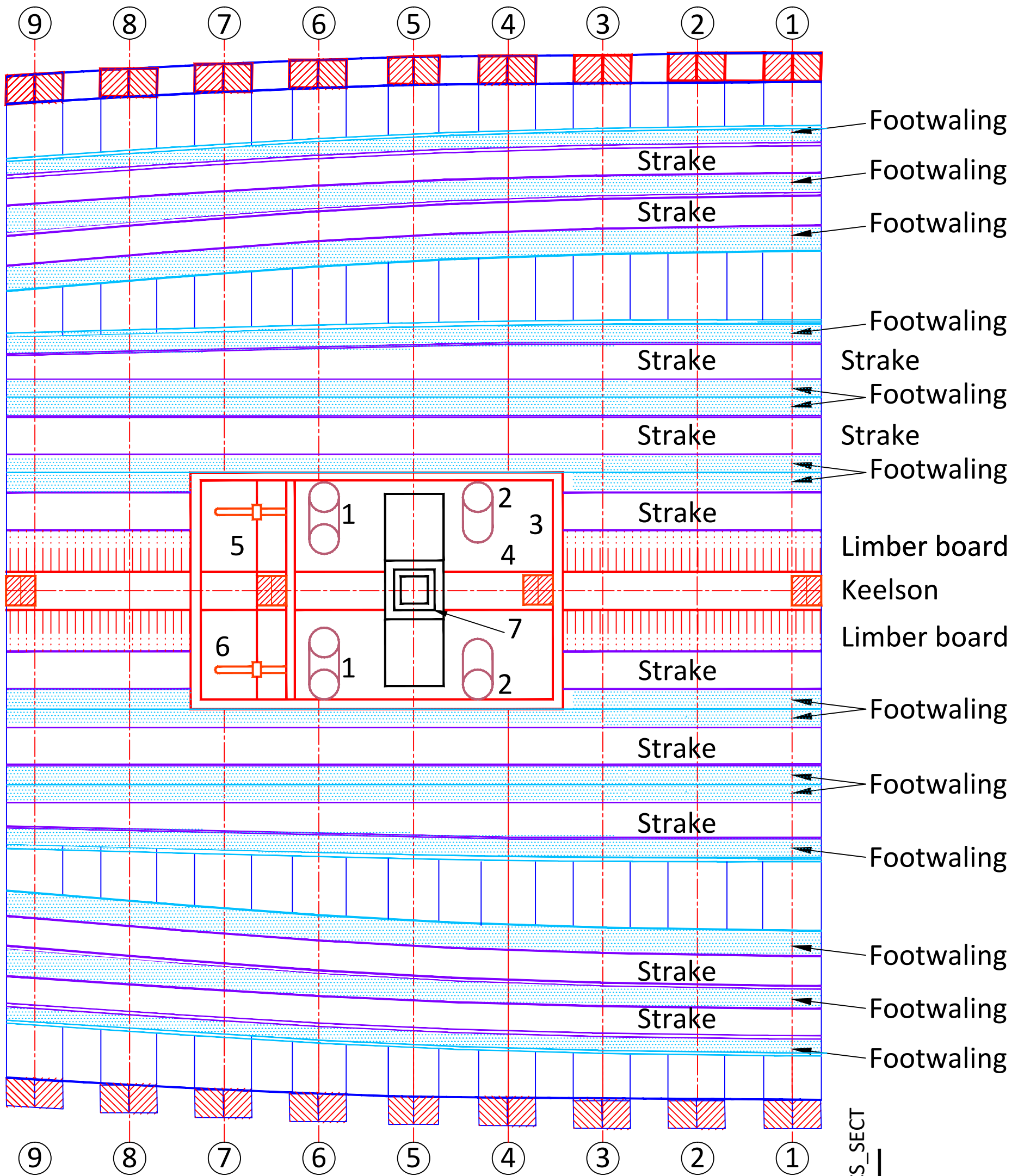
Hold Plan 1:32
