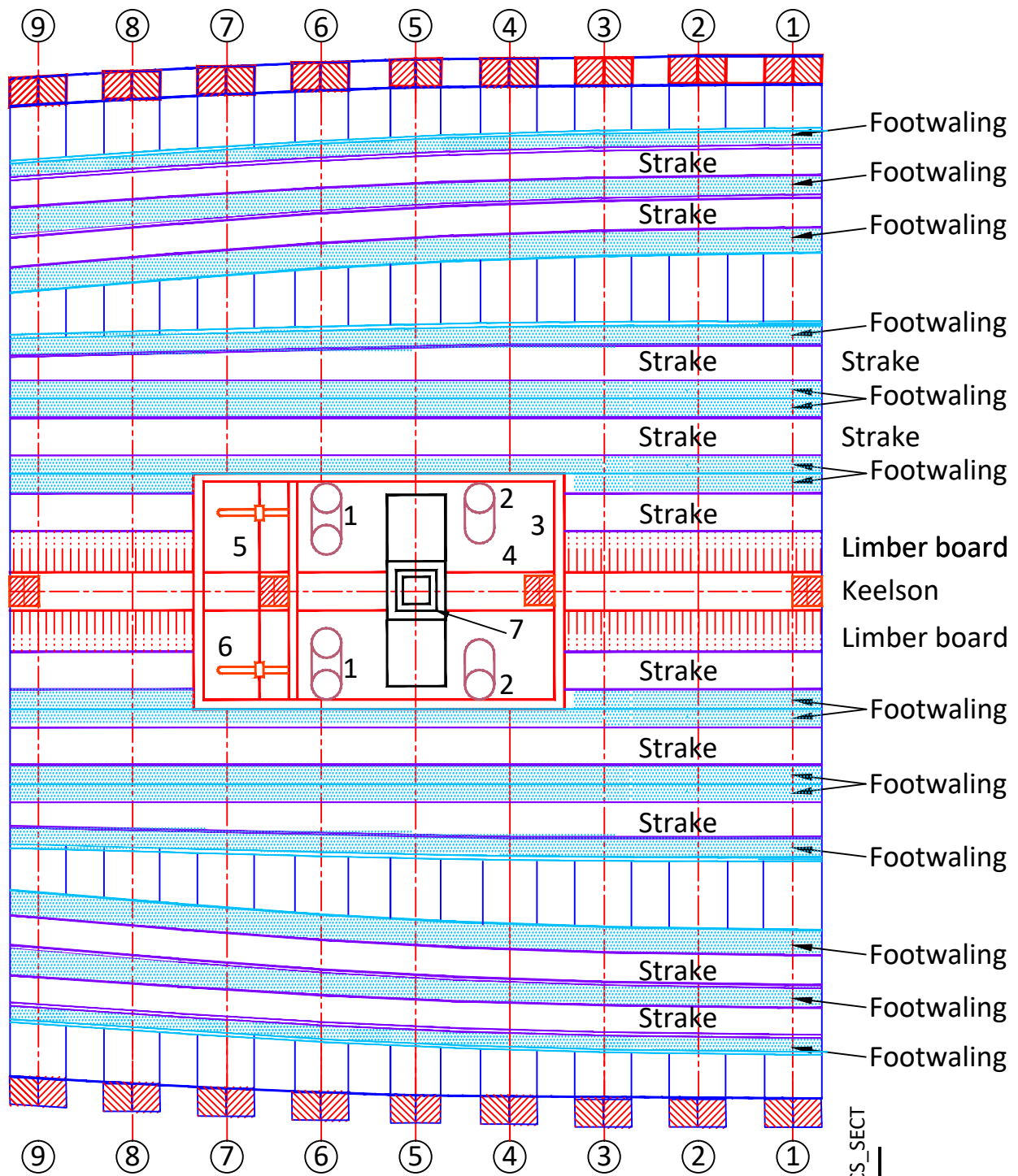
Hold Plan 1:48
